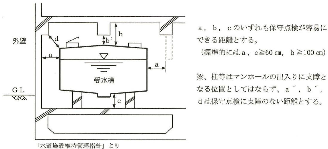
図－4．26 受水槽設置断面図
