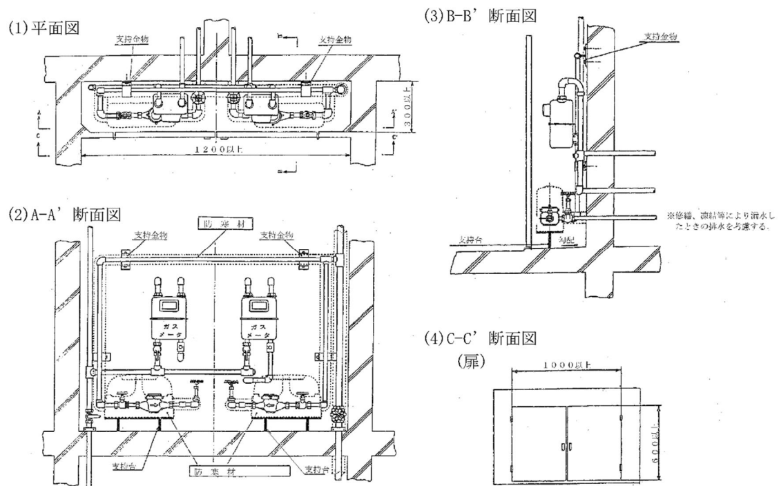
図－４．１９ メーターボックス及び扉の標準寸法 (メーター２個並列の場合)
