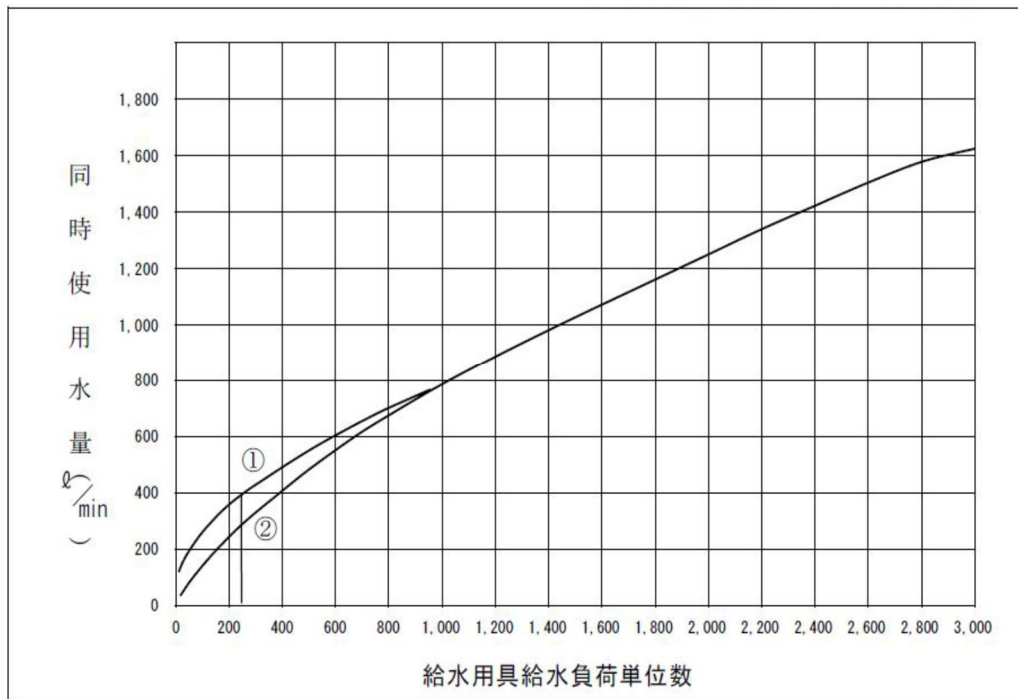
図－ 4． 1 同時使用水量図（空気調和衛生工学便覧参考）
