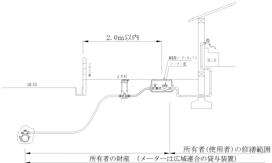
図一 7. 1 給水装置の漏水修繕区分図
