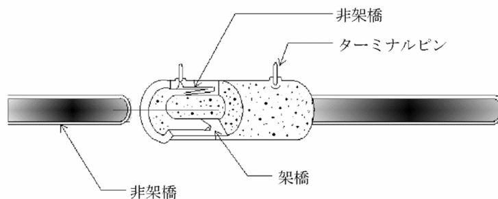
図－５．９ 電気式熱融着継手【E種】
