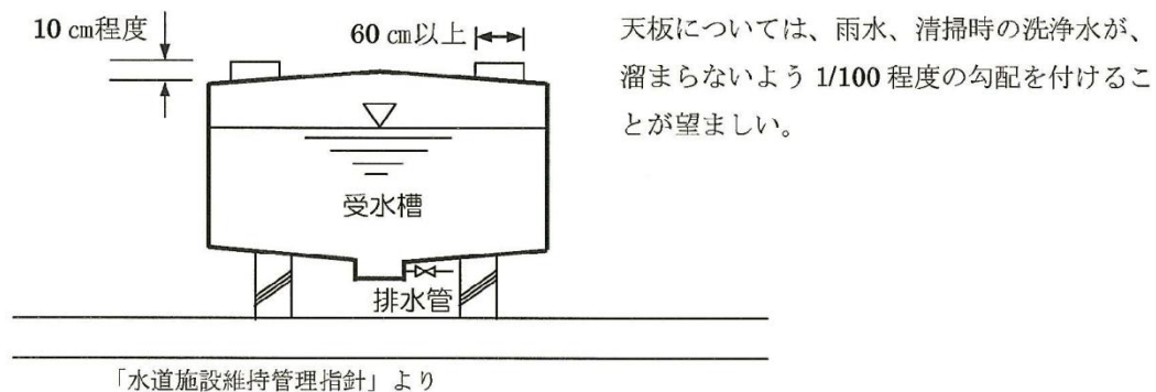
図－4．27 マンホール及び排水管の設置
