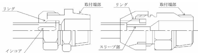
図－５．８ メカニカル継手【M種】
