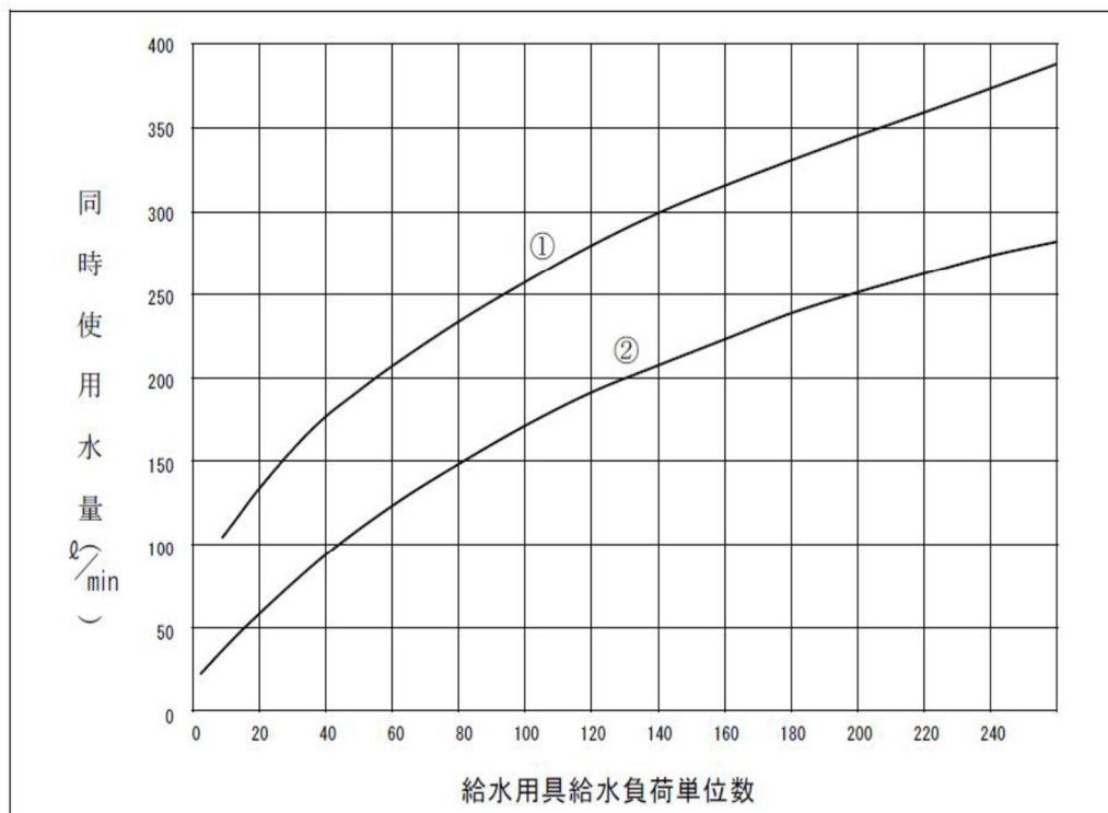
図－ 4． 2 同時使用水量図（拡大図）
