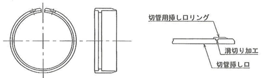
図－５．２２ 切管用挿しロリング
