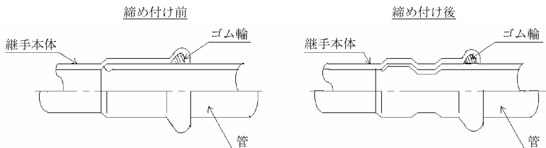
図－５．１４ プレス式継手
