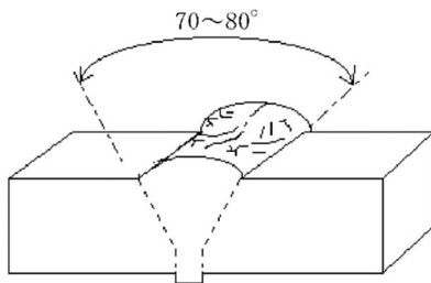
図－５．２５ V型開先
