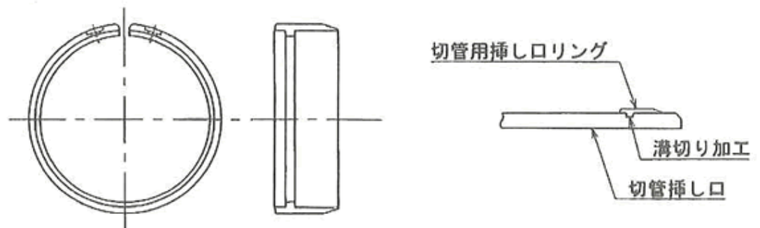
図－５．２２ 切管用挿し口リング
