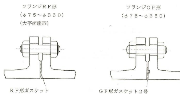
図－５．２３ フランジ接合
