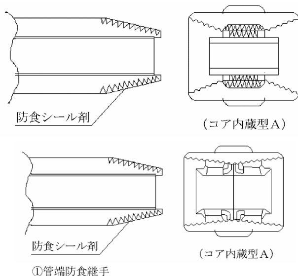
図－５．５ ねじ接合
