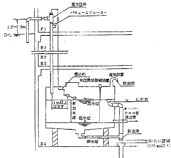
図－４．３３ 受水槽設置標準図（４）
