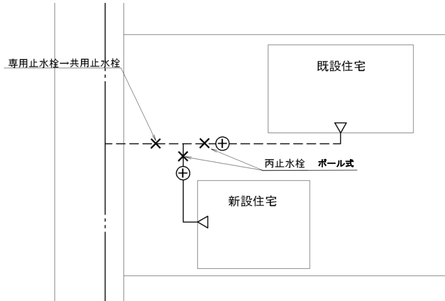
図－４．１１ 既設給水管からの分岐 (既設給水管に給水能力がある場合)
