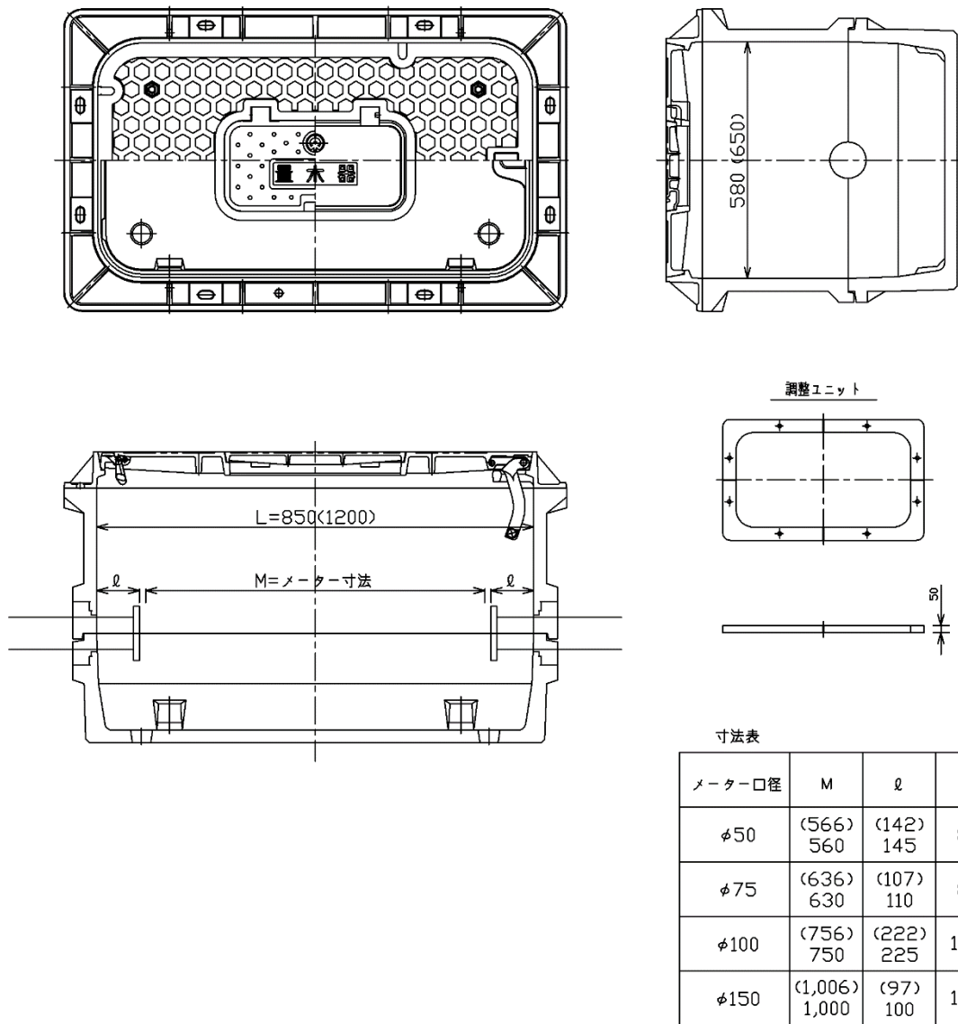
図-4. 16 メーターボックス構造図 (大型メーターユニット)
