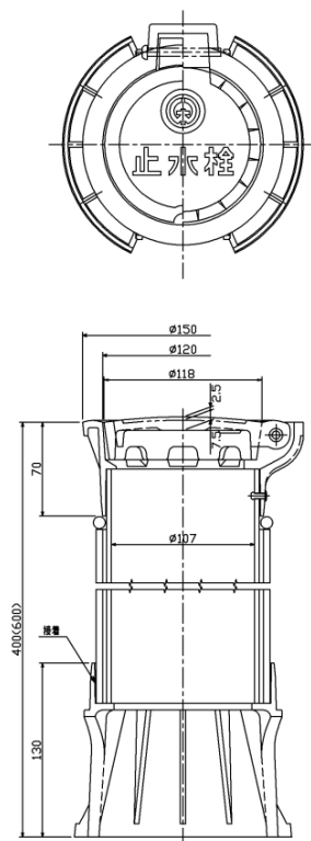
止水栓筐 (宅内用)
