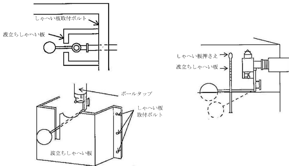
図－４．２９ ボールタップ式受水槽
