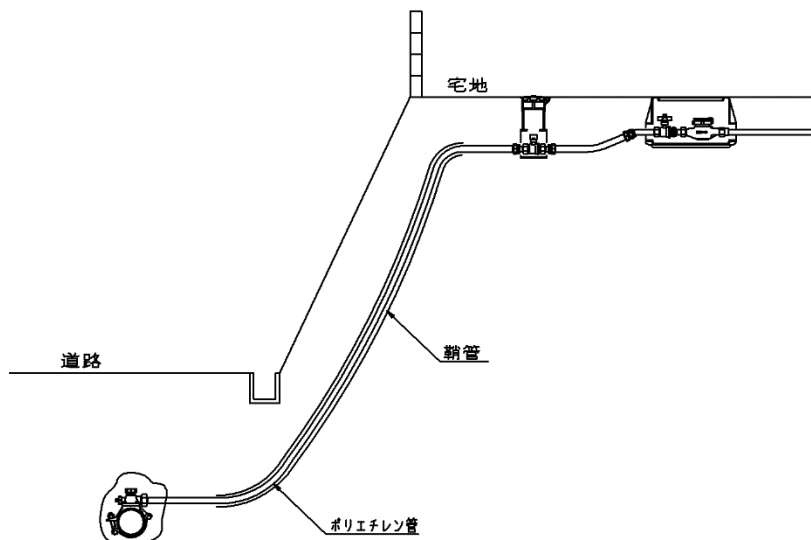
図－４．２４ さや管図
