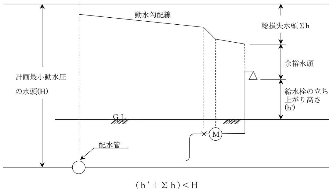
図－4.3 水頭変化曲線
