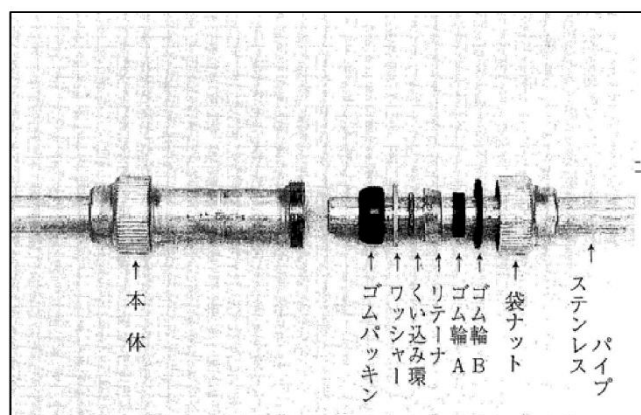
図－５．１３ 伸縮可とう式継手の接合
