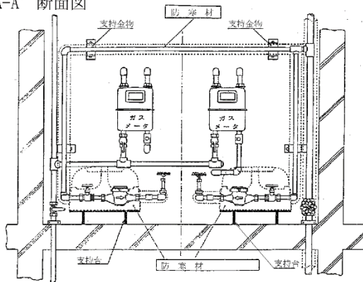
(2) A-A' 断面図
