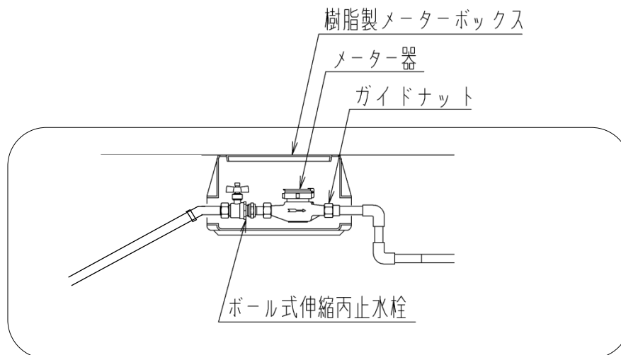
図－４．１５ メーターボックス
