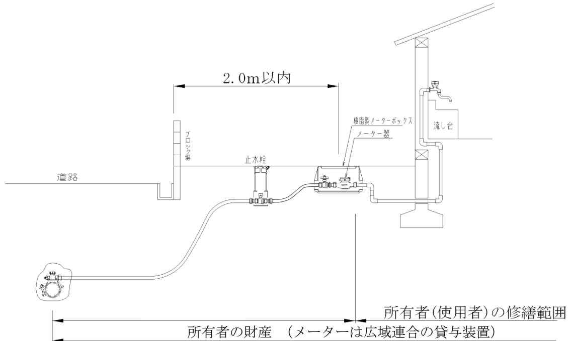
図ー 7. 1 給水装置の漏水修繕区分図
