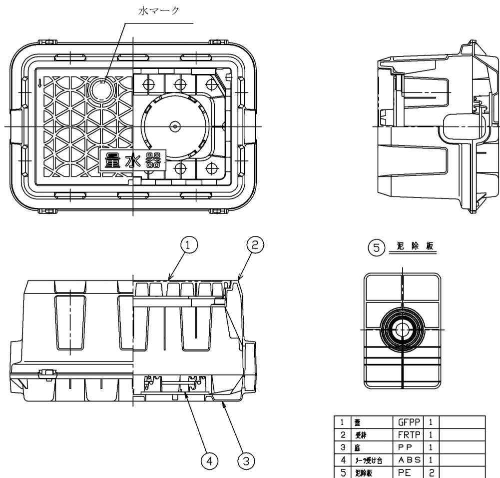
図－４．１４ メーターボックス
