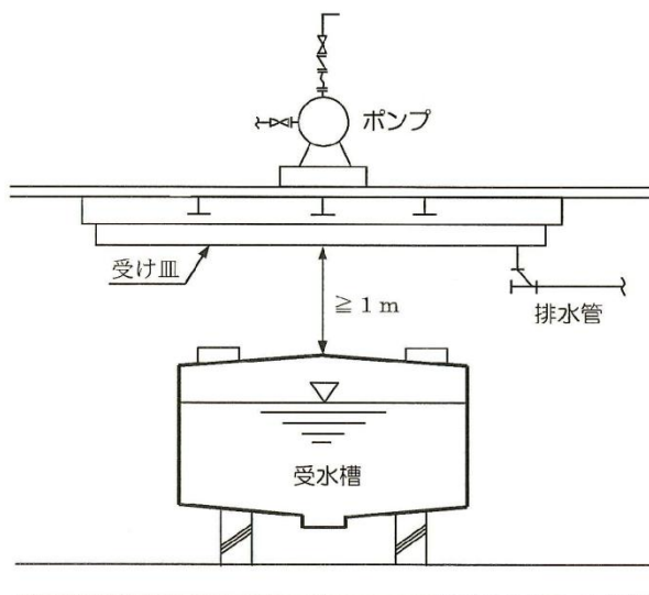
図－４．２８ 受水槽上部に機器類を設置した場合
