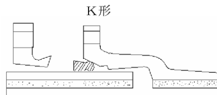
図－５．１８ メカニカル継手（K形）の接合
