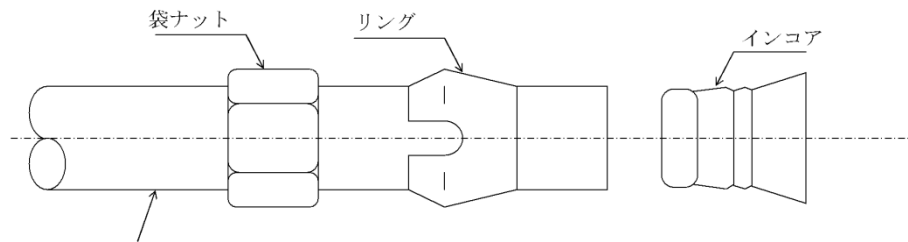
図－５．６ メカニカル継手の接合
