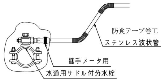
図ー 4. 2 2 ( 2 ) 給水装置施工図 ステンレス鋼管 ( 2 5 mm 以下)
