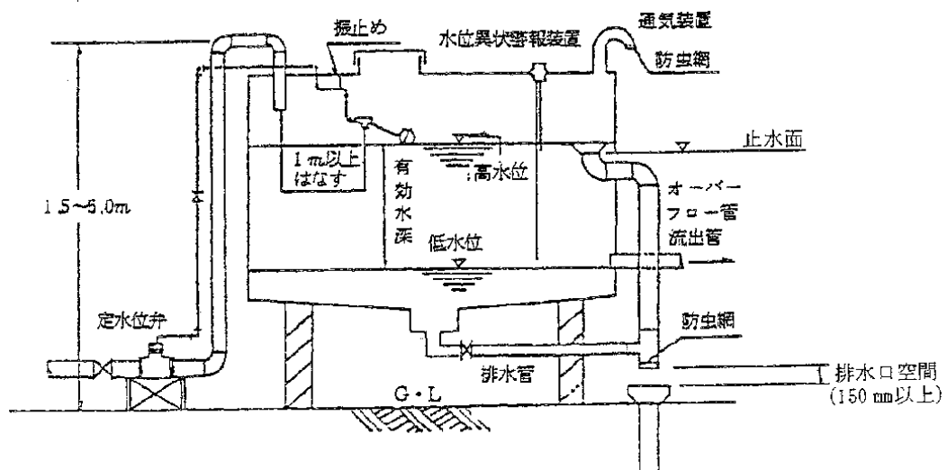
図－４．３１ 受水槽設置標準図 (2)
