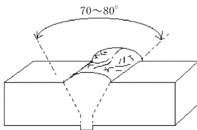
図－５．２５ V型開先
