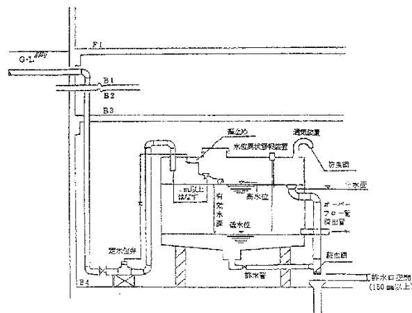
図－４．３３ 受水槽設置標準図（４）
