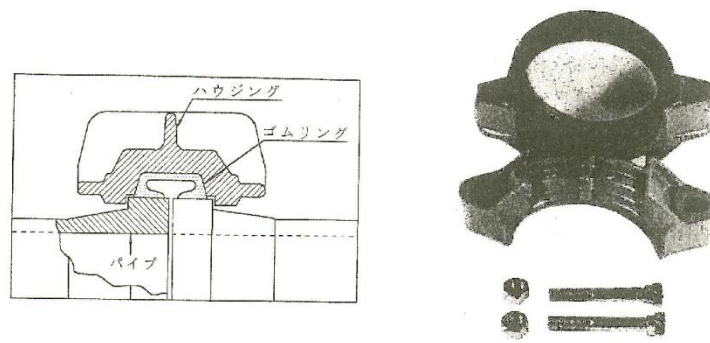
ビクトリック継手
