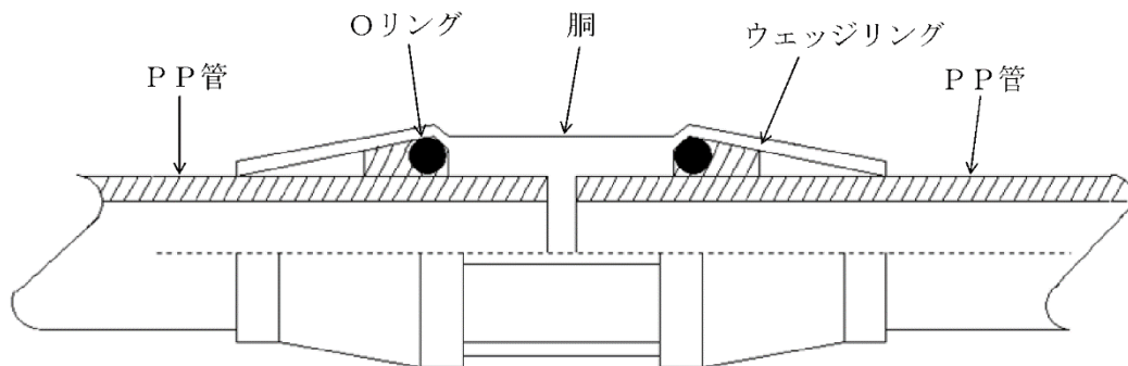
図－５．７ ワンタッチ式継手
