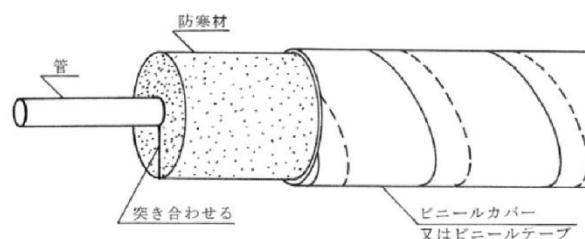
図－6．3 防寒措置
