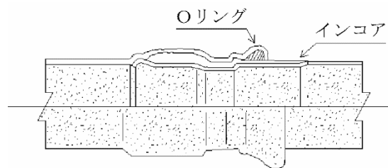
図－５．１７ プレス式接合
