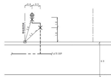
オフセット図 S=Free
