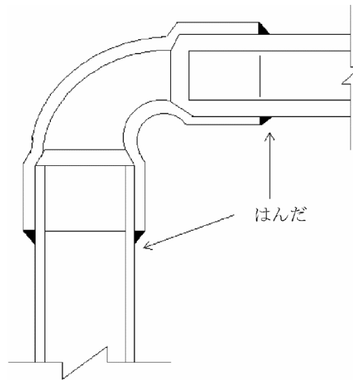
図－５．１６ はんだ接合
