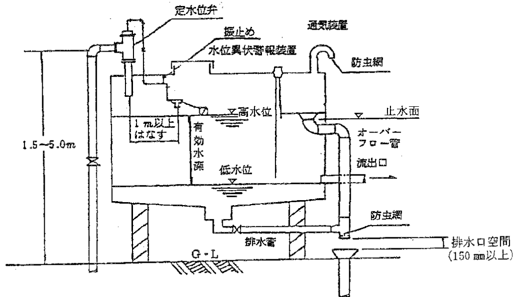
図－４．３０ 受水槽設置標準図 (1)
