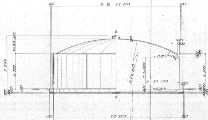
立面図 S=1/50
