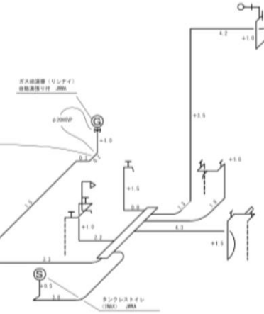
立面図 S=Free
