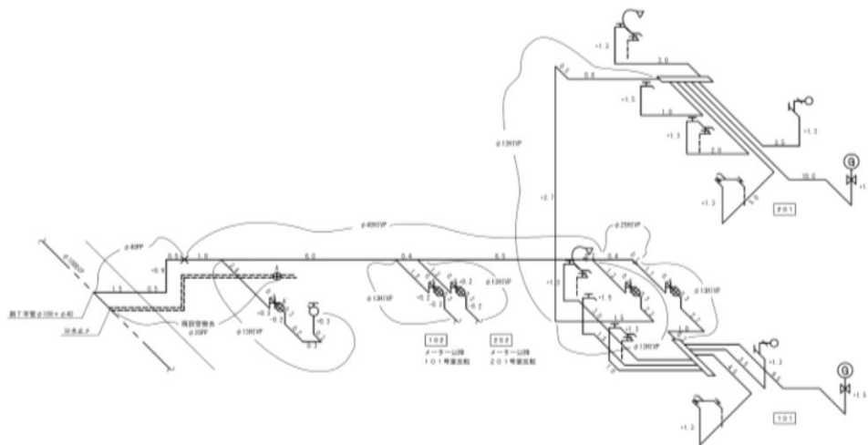
立面図 S=FREE
