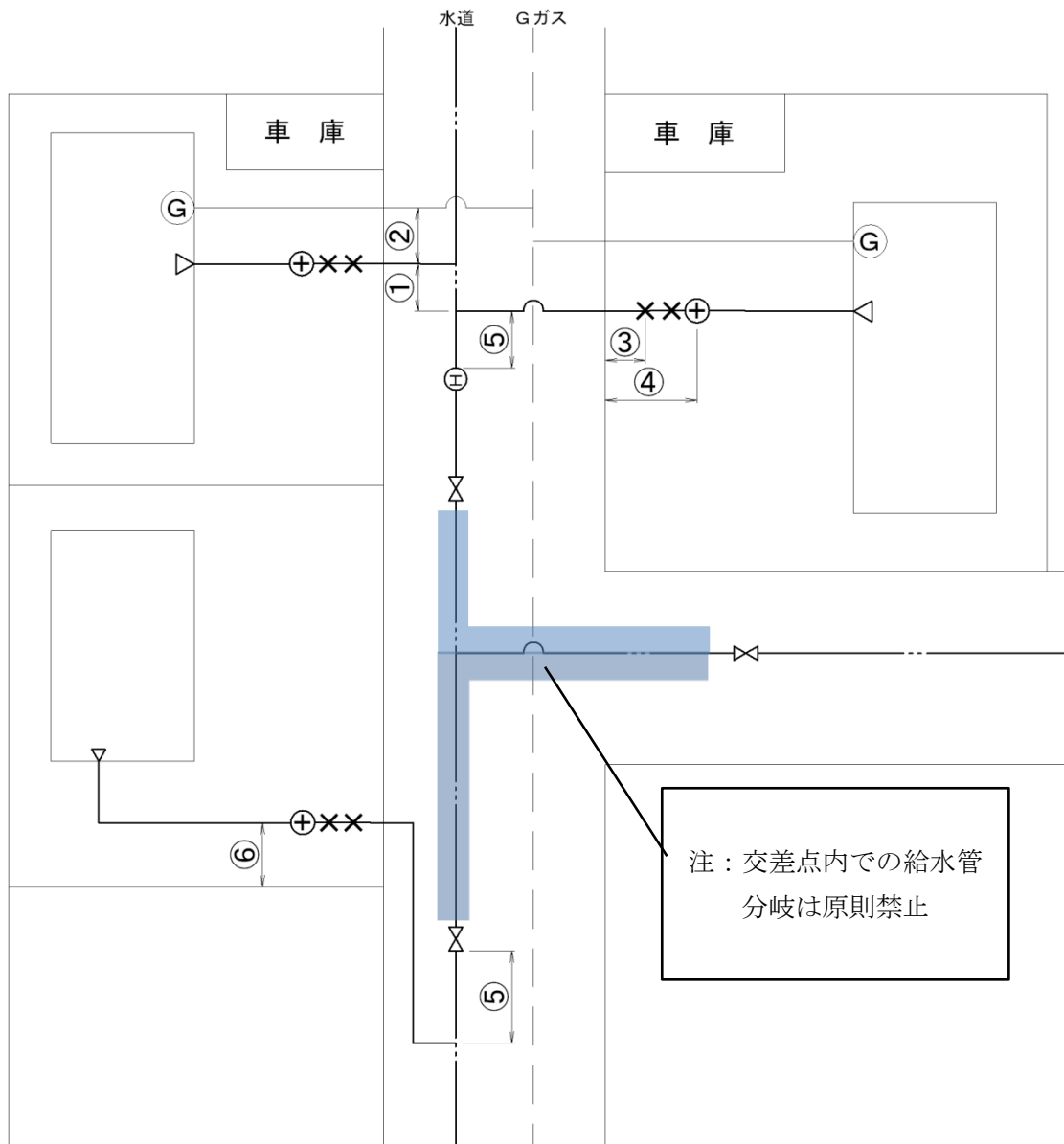
図-4.6 取り出し標準図1
