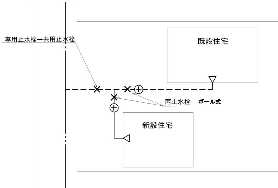
図ー 4. 1 1 既設給水管からの分岐 (既設給水管に給水能力がある場合)
