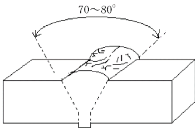
図-5. 25 V型開先
