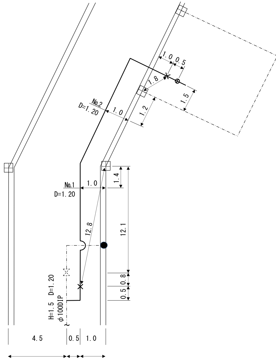
オフセット標準図 S=free (例3)
