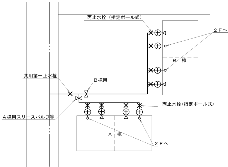
図-4.8 取り出し標準図3
