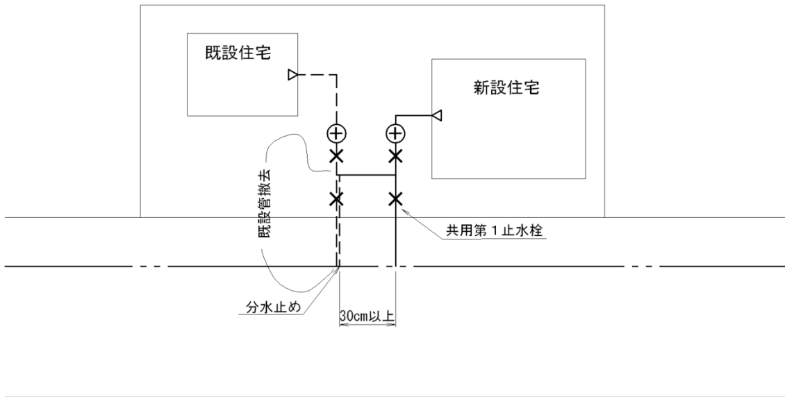
図-4.10 既設給水装置がある場合 (既設給水管の給水能力が不安な場合)
