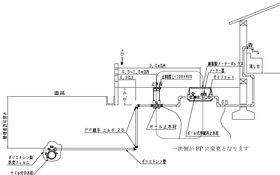
口径25mmポリエチレン管取出し標準図(直角取出し)
