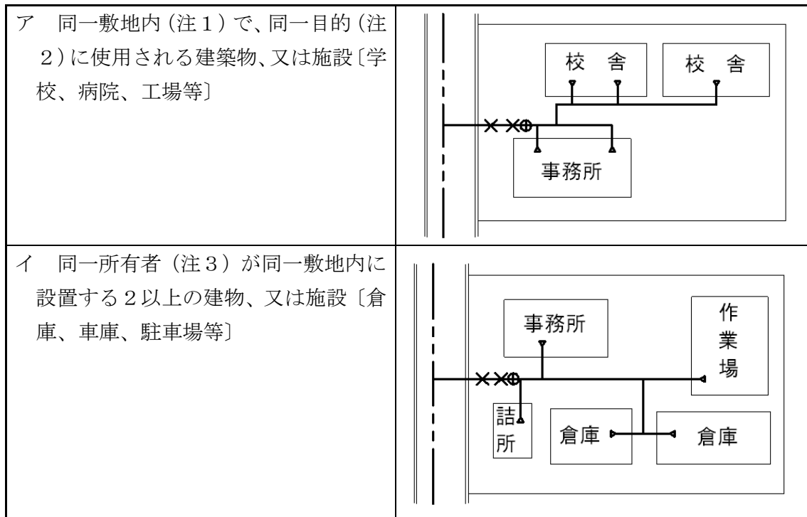
図：標準図
