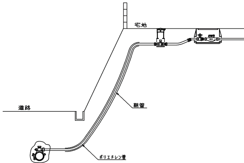
図-4.24 さや管図
