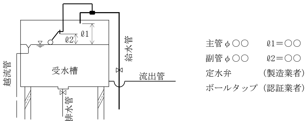
吐水口空間図
