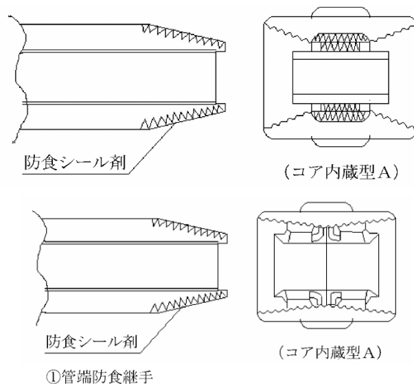
図-5.5 ねじ接合
