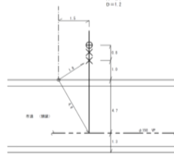
オフセット図 S=Free
