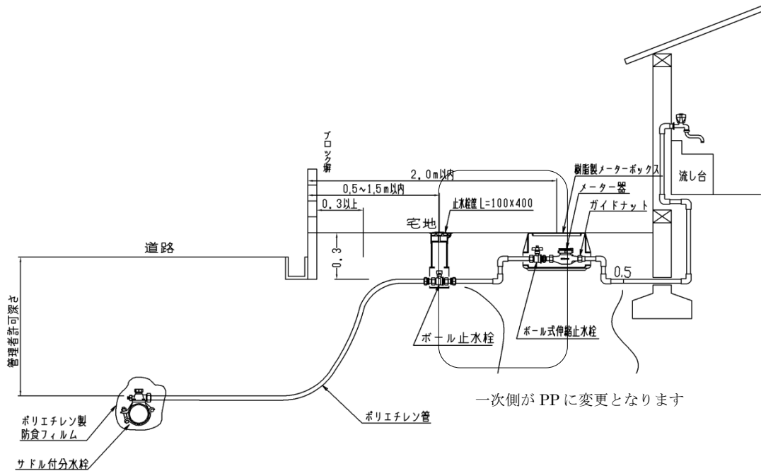
図-4.21(1) 給水装置施工図 口径20mmポリエチレン管取出し標準図(直角取出し)
